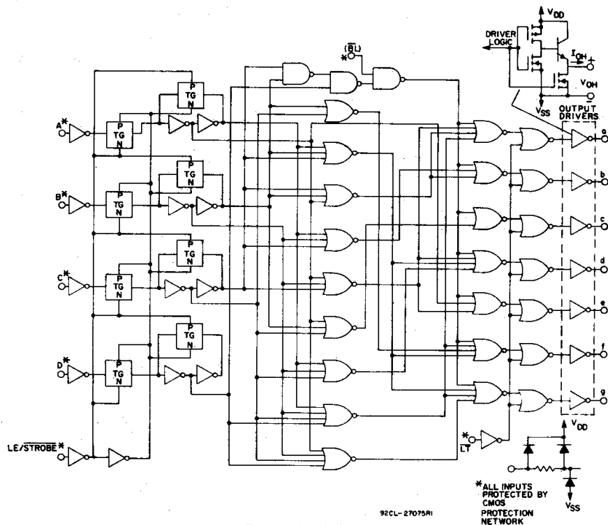
Fig. 8 - Logic diagram.
