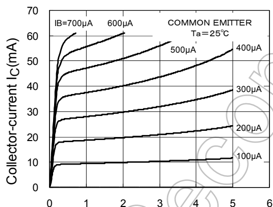
I_C-V_{CE}
