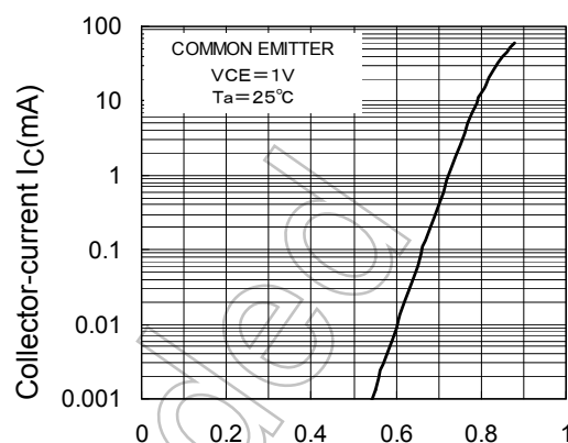
I_C-V_{BE}
