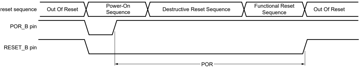
Figure 17. POR due to POR_B pin assertion
