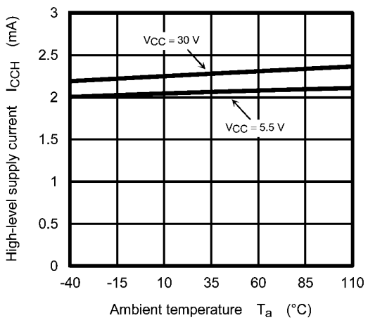
Fig. 12.2.8 I_{cCH} - T_a
