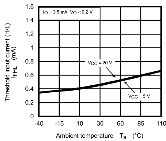
Fig. 12.2.2 I_{FHL} - T_a
