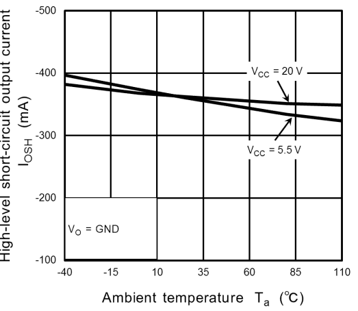
Fig. 12.2.10 I_{osH} - T_a
