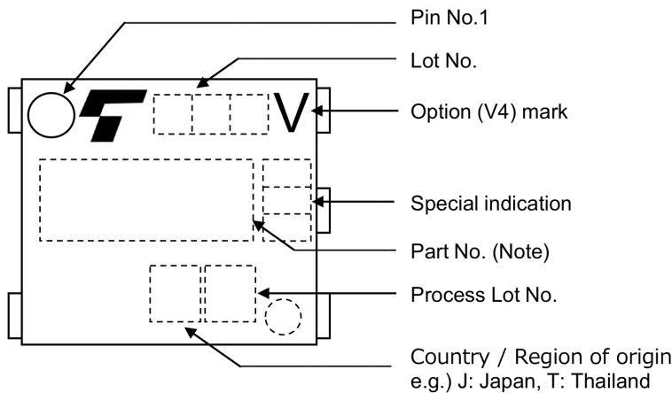
Fig. 16.4 Marking Example(Note)
