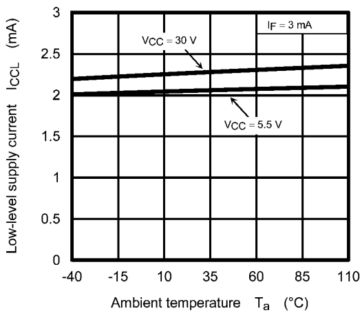
Fig. 12.2.7 I_{cCL} - T_a
