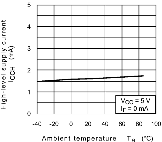
Fig. 13.2.6 I_{CCH} - T_a
