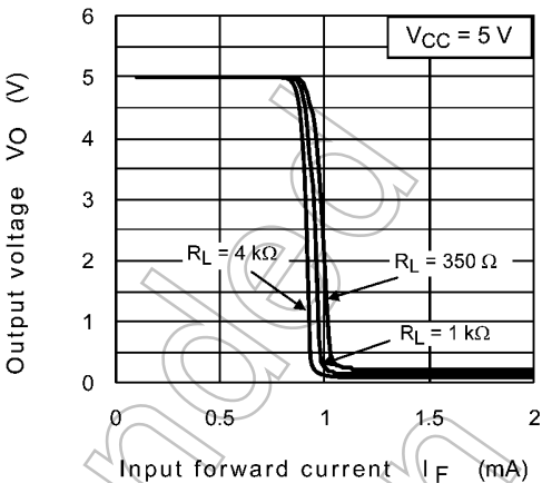
Fig. 13.2.2 V_O - I_F
