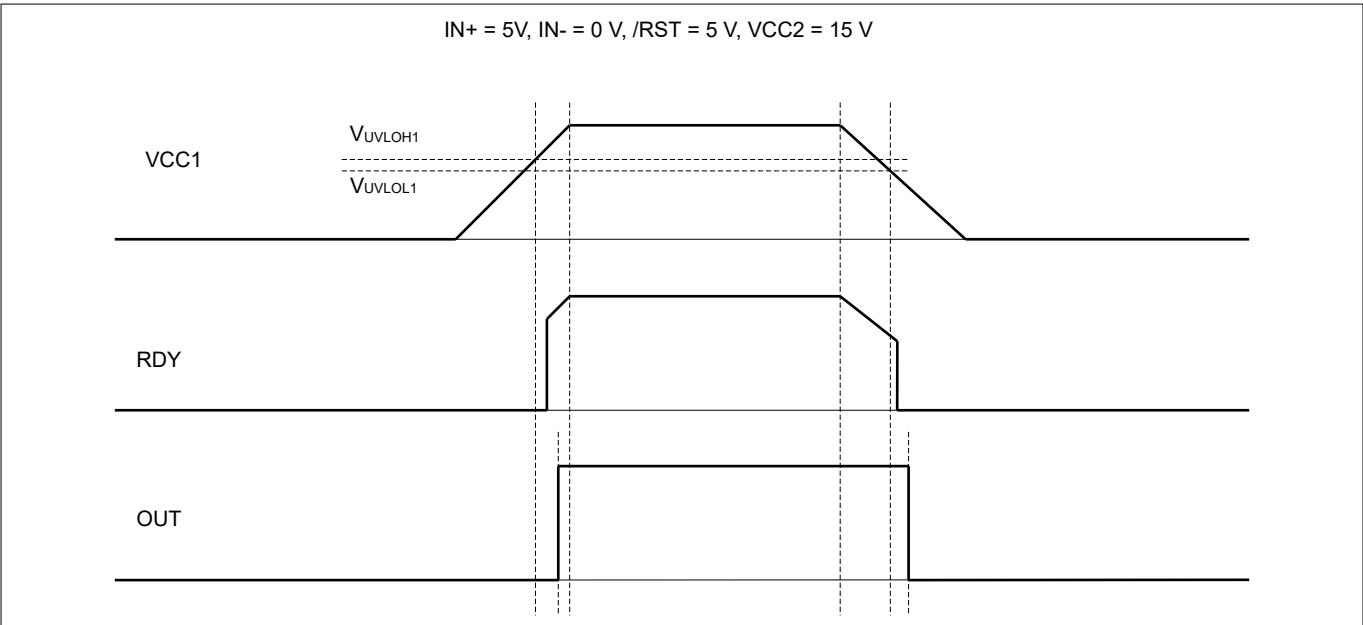
Figure 8 UVLO1
