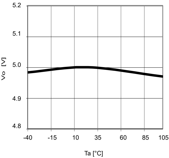
Fig.21 T_a-V_O (I_o=0mA)
