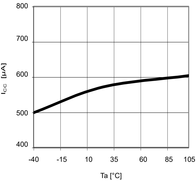
Fig.22 T_a-I_{CC}
