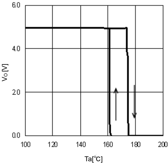
Fig.28 TSD ( I_o=0\text{mA} )
