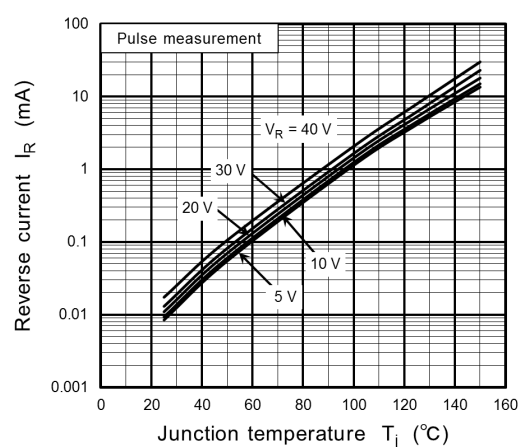
Fig. 10.8 I_R - T_j
