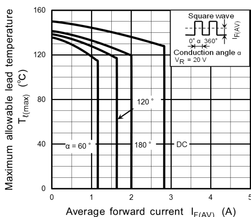
Fig. 10.4 T_{l(max)} - I_{F(AV)}
