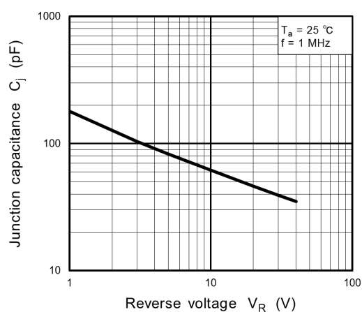
Fig. 10.7 C_j - V_R
