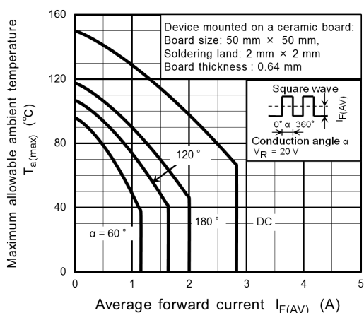
Fig. 10.3 T_{a(max)} - I_{F(AV)}
