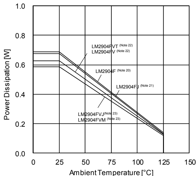
(d) LM2904xxx
