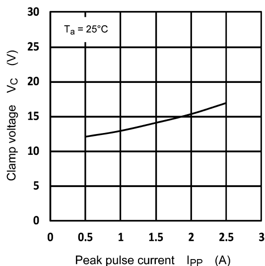
Fig. 9.1 V_C - I_{PP}
