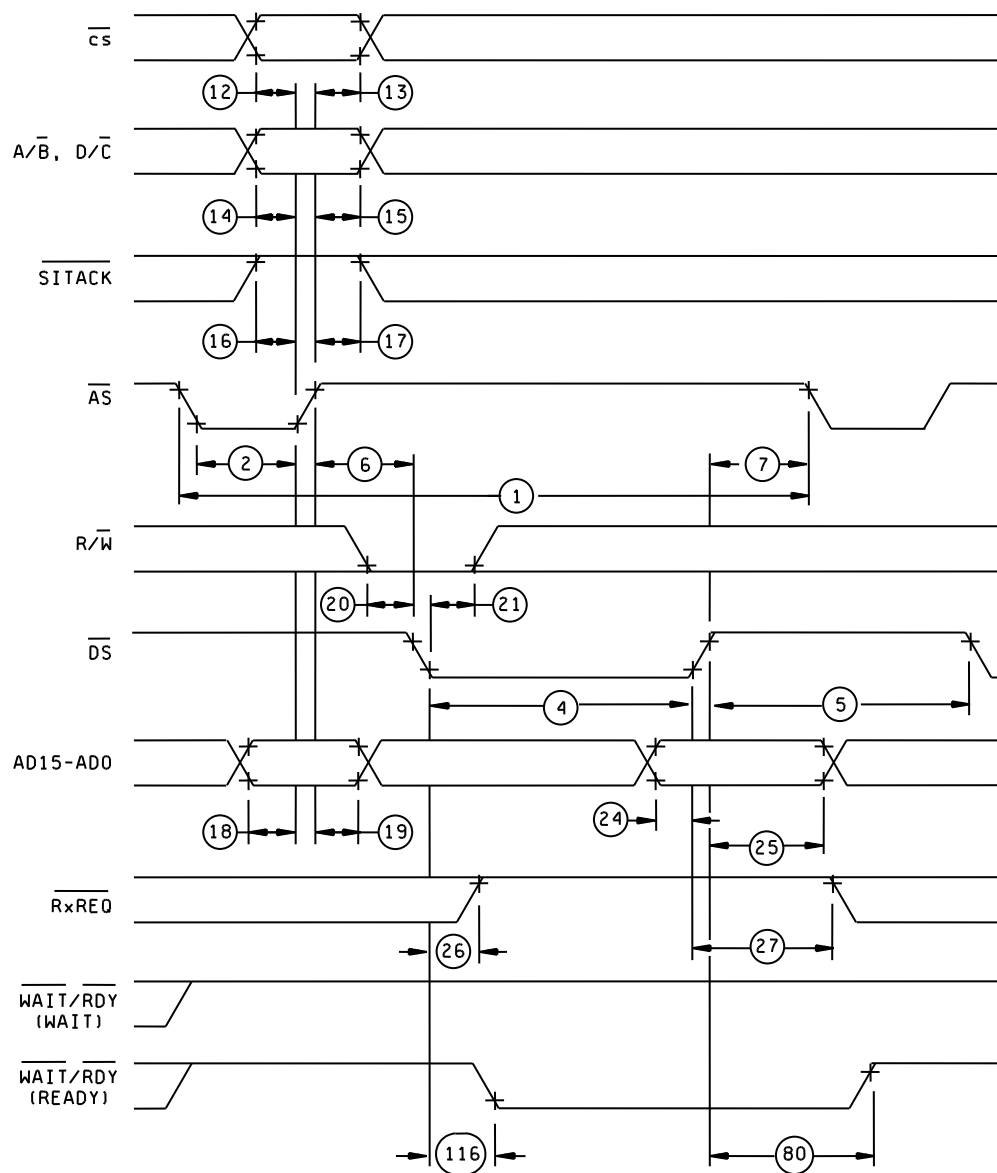
MULTIPLEXED DS WRITE CYCLE
