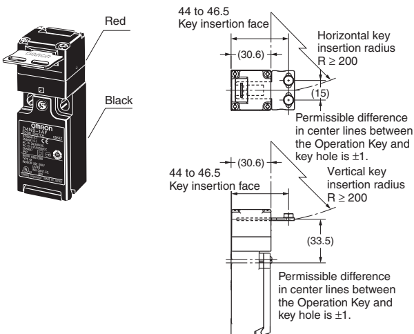
D4NS-1□F + D4DS-K3
