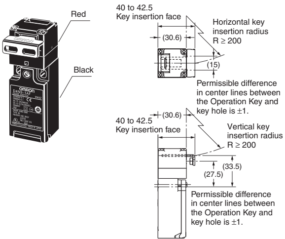
D4NS-1□F + D4DS-K5
