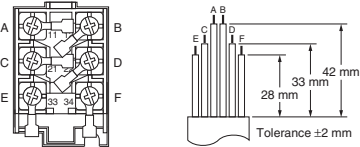
(2 conduits type)
