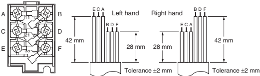
(2 conduits type)
