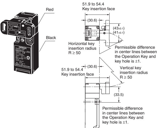
D4NS-1□F + D4DS-K5
