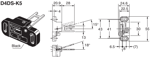
D4DS-K5
