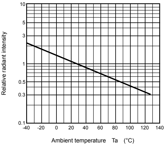
Relative I_E - Ta (typ.)
