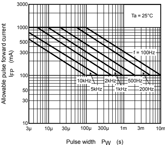
I_{FP} - P_W
