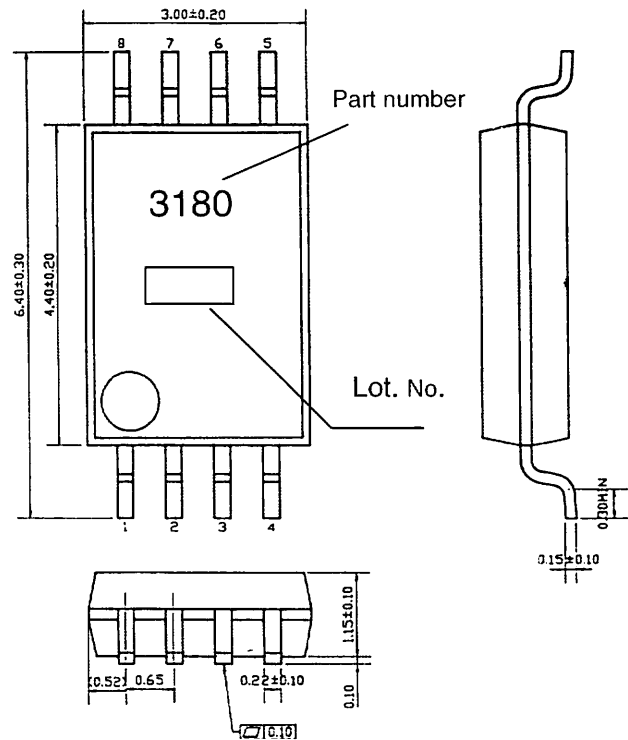
SSOP-B8 (UNIT : mm)
