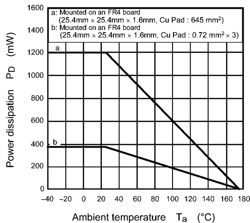
Fig. 9.13 P_D - T_a
