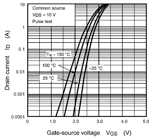
Fig. 9.2 I_D - V_{GS}
