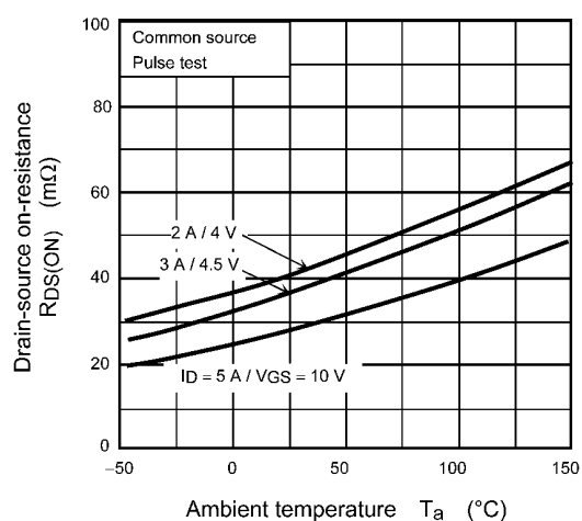
Fig. 9.5 R_{DS(ON)} - T_a
