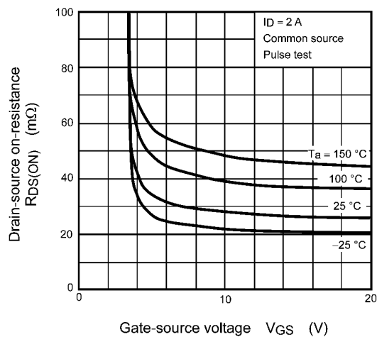
Fig. 9.3 R_{DS(ON)} - V_{GS}
