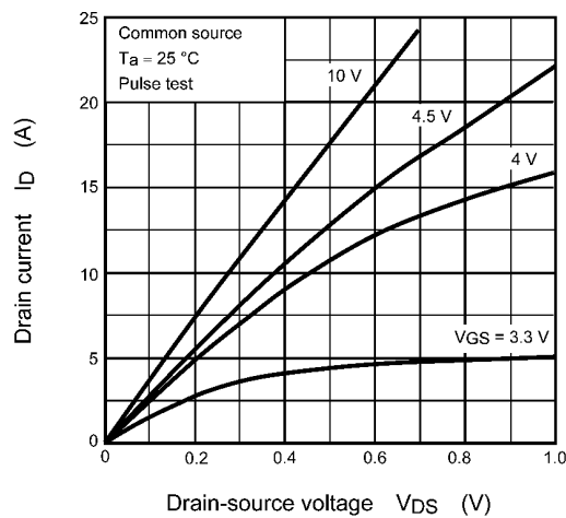
Fig. 9.1 I_D - V_{DS}
