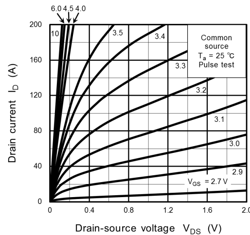
Fig. 8.2 I_D - V_{DS}
