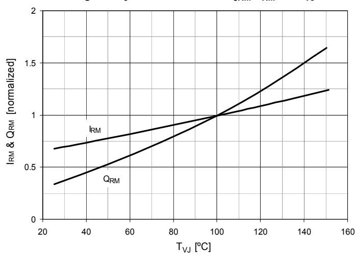
Fig. 25. Dynamic Parameters Q_{RM} , I_{RM} vs. T_{VJ}
