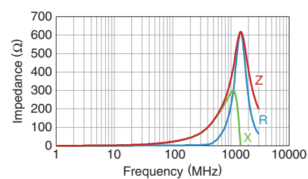
MMZ0603F220CTD25
