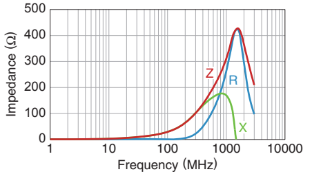
MMZ0603D800CTD25
