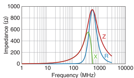
MMZ0603D121CTD25
