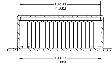
SECTION D-D
