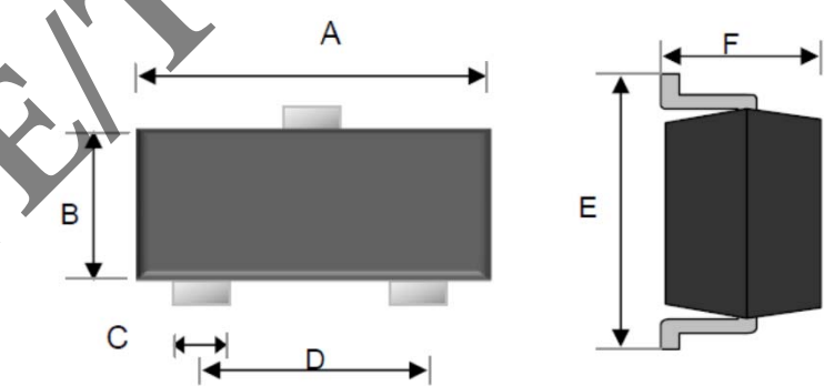
SOT-723
