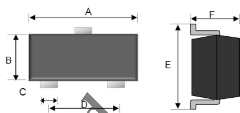
SOT-323
