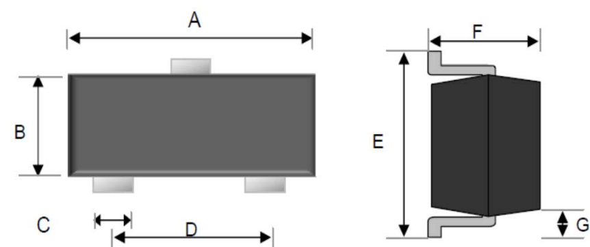
SOT-23
