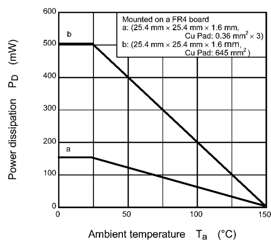
Fig. 7.13 P_D - T_a
