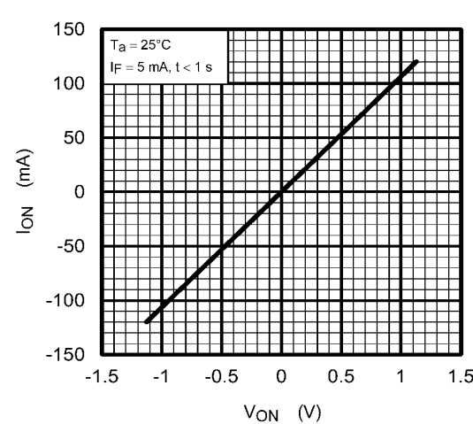
Fig. 12.4 I_{ON} - V_{ON}
