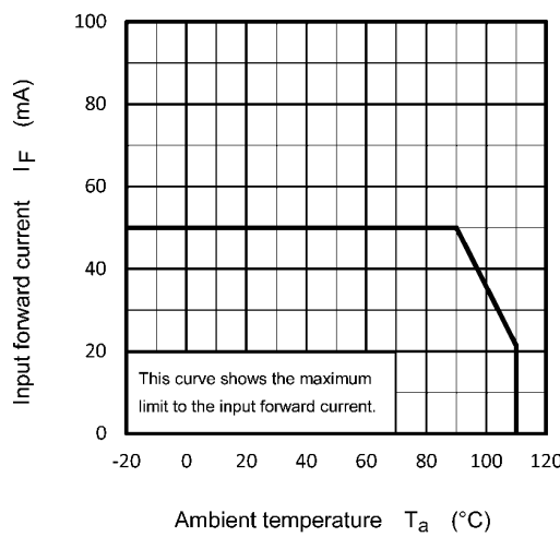
Fig. 11.1 I_F - T_a
