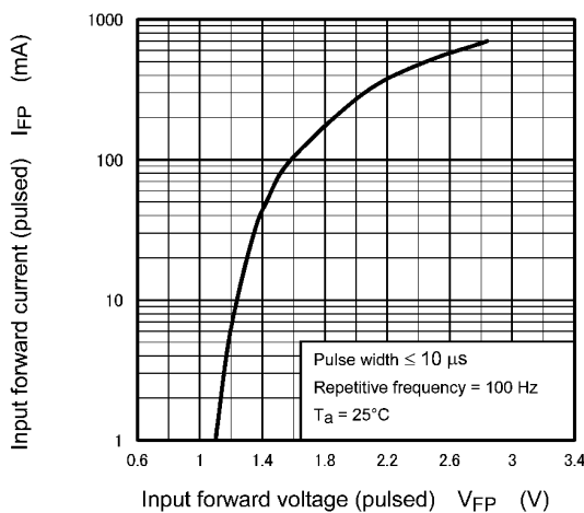
Fig. 11.6 I_{FP} - V_{FFP}
