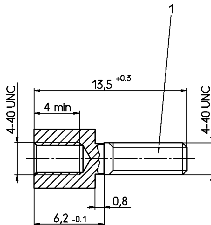
Sechskant SW 4,5
