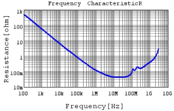
GCJ32DR72J223KXJ1 R DCOV, 25degC
