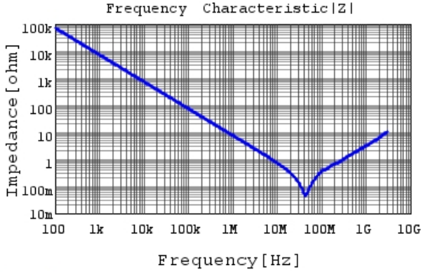
GCJ32DR72J223KXJ1 |Z| DCOV, 25degC
