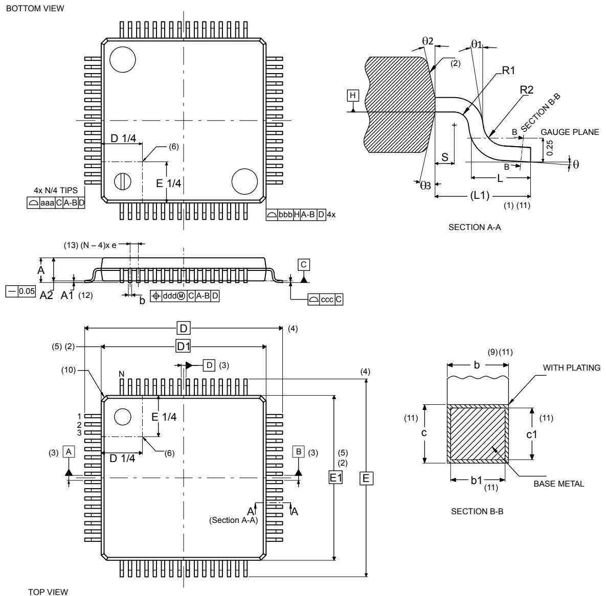
Figure 45. LQFP64 - Outline (15.)
