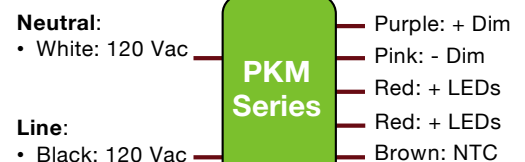
Wiring Diagrams
