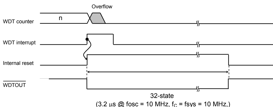
Fig. 16-3 Reset Mode
