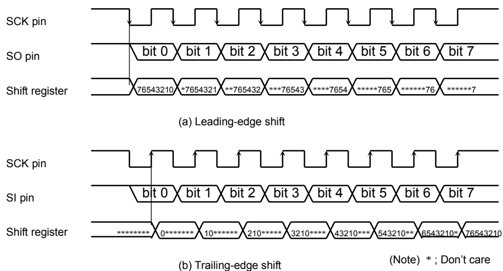
Fig. 12-26 Shift Edge
