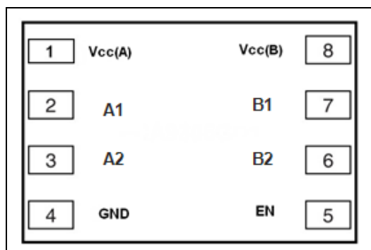
UDFN Package
