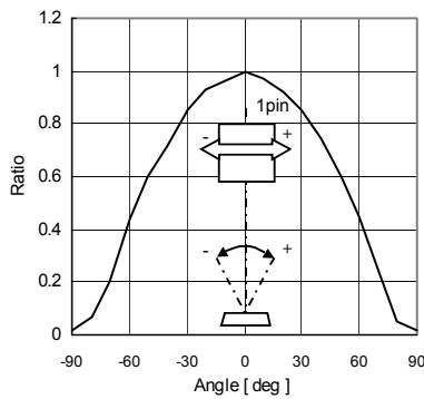
Fig.4 ALS Directional Characteristics 1
