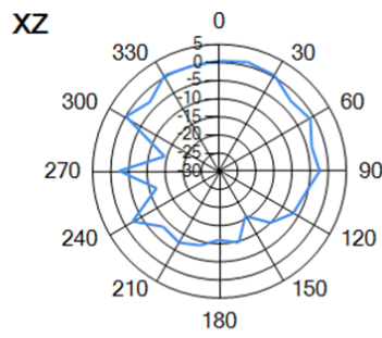
— 6.55GHz
