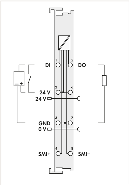
SMI Master LoVo; 24 VDC
