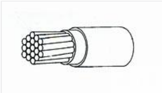
TE Part #218562-000 22759/34-22-0
