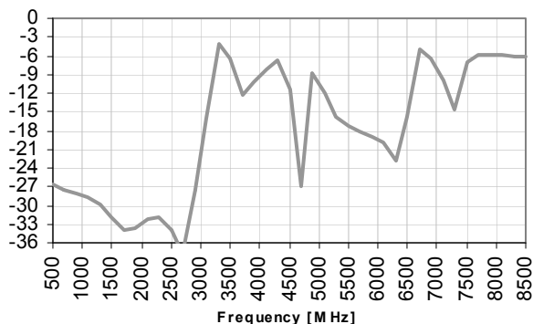
CMRR
