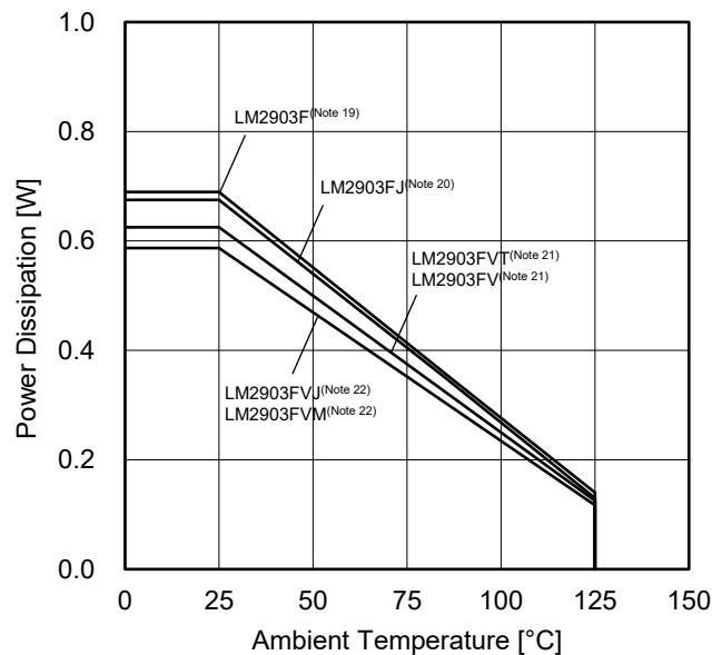
(d) LM2903xxx*2
