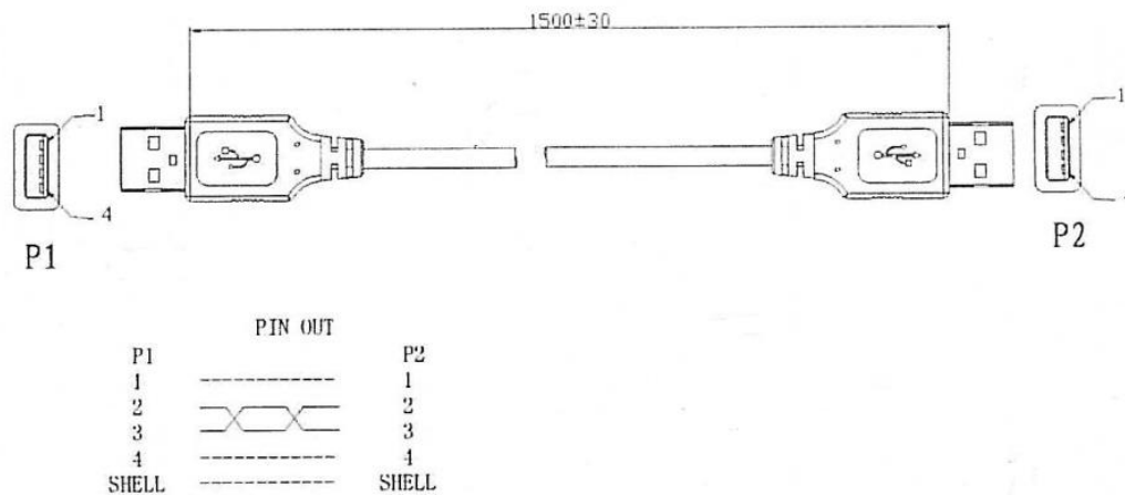
USB CABLE
