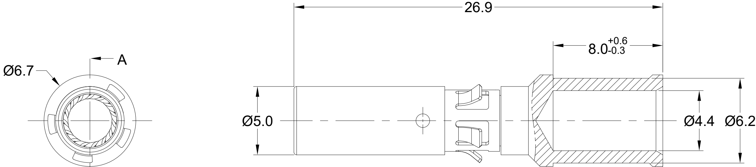
SECTION A-A
